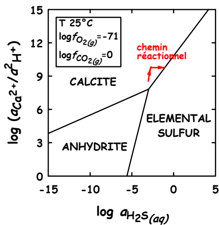
Figure 3 : Domaines de stabilité de la calcite, de l'anhydrite et du soufre élémentaire à 25 °C, pour une fugacité de CO 2 gaz de 1 bar et des fugacités d'oxygène fixées par l'assemblage pyrite-pyrrhotite-magnétite. Les flèches indiquent le chemin réactionnel.
