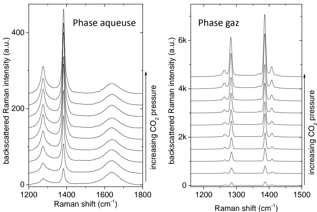
Figure 9 : Spectres de diffusion Raman enregistrés dans la phase aqueuse et la phase gaz à l'aide des sondes à immersion à 100^\circ\text{C} et à des pressions variant régulièrement de 10 à 200 bar. Les spectres sont centrés sur les bandes du \text{CO}_2 .
