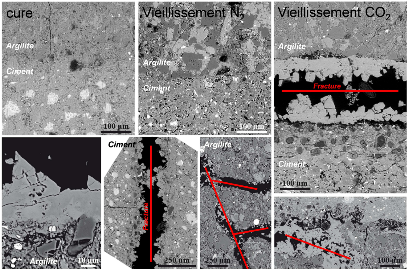
Figure 14 : Résultats de l'expérience « sandwich » décrivant le comportement de l'interface argilite/ciment après cure (7 jours à 100 bar de N_2 et 80^\circ C ), après vieillissement à l'azote ou après vieillissement au CO_2 en phase aqueuse (30 jours à 110 bar et 80^\circ C ). L'expérience montre très clairement l'influence du CO_2 et de la carbonatation sur l'ouverture de l'interface et sur la fracturation de l'argilite. Ces résultats doivent être interprétés en terme d'intégrité des puits d'injection au voisinage de la couverture. Thèse Emmanuel Jobard et projet ANR Interface.
