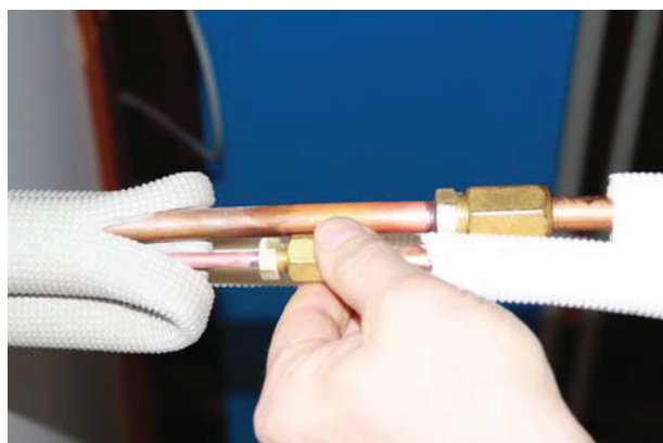
14. Koppelingen op binnendeel voorzichtig handvast draaien en daarna passende sleutels vastdraaien
