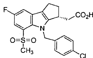
Jedinjenje E
