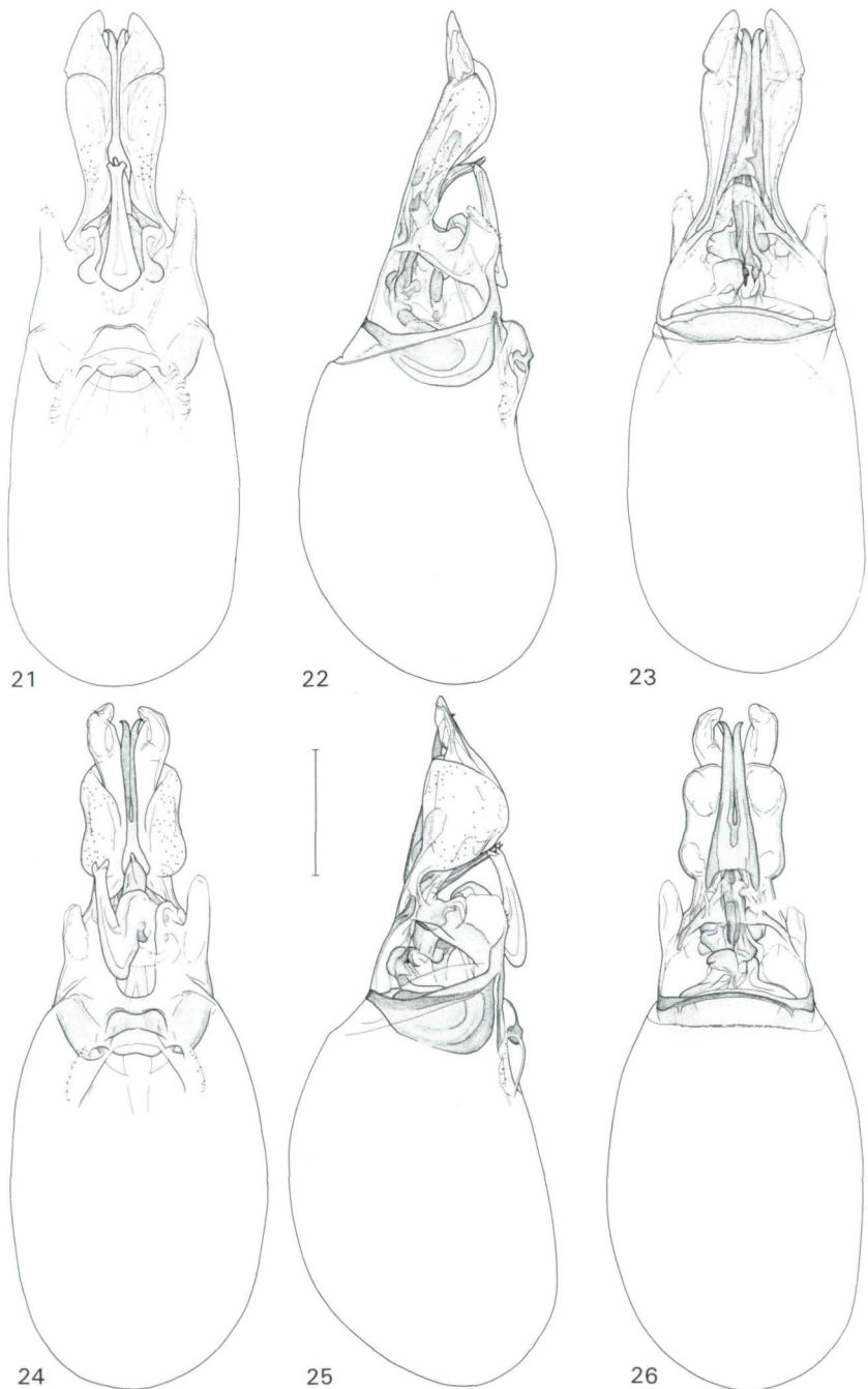
Figs. 21-23: Scopaeus franzi , ♂, Portugal, Vila Real: aedeagus in 21) ventral, 22) lateral, 23) dorsal view. Figs. 24-26: S. hispanicus , ♂, Spain, Burgos: aedeagus in 24) ventral, 25) lateral, 26) dorsal view. Scale bar = 0.1 mm.
